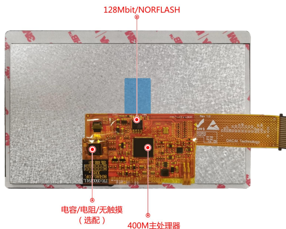
图 1-4 硬件配置图
