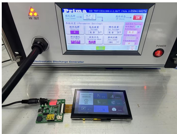
图 7-2 ESD 测试图
